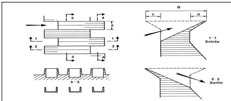
Fig. 8. P.K.Weir à porte-à-faux amont et aval identiques (Type A)
