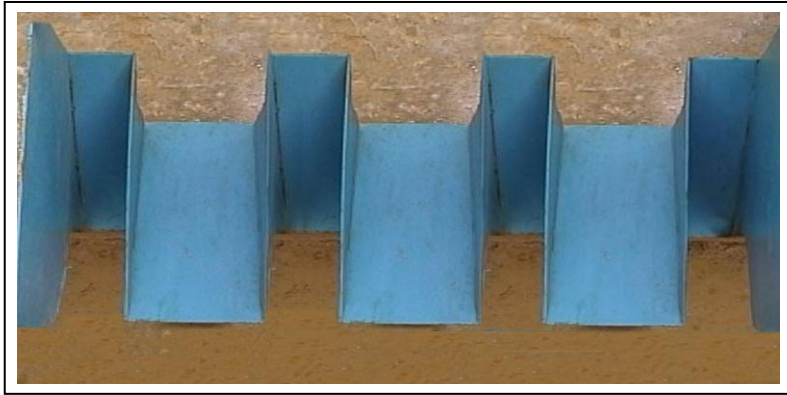
Fig. 3. Vue en plan du modèle réduit du P.K.Weir
