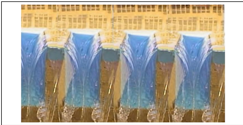
Fig. 4. Vue aval de l'écoulement sur le P.K.Weir
