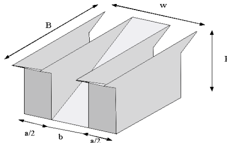
Fig. 1. Schéma d'un cycle de déversoir en clefs de Piano (P.K.Weir)
