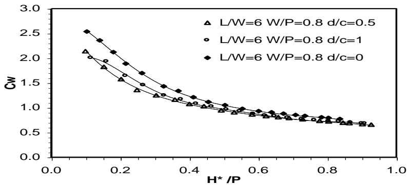
Fig. 7. Coefficient de débit du P.K.Weir en fonction de la longueur des porte-à-faux
