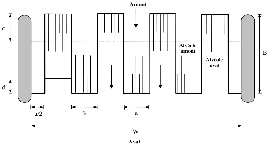
Fig. 2. Vue en plan du déversoir en clefs de Piano (P.K.Weir)
