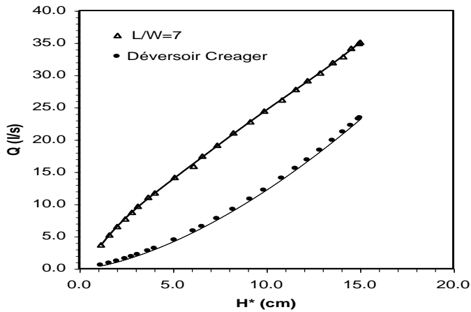
Fig. 5. Comparaison entre le débit évacué par le P.K.Weir et celui d'un déversoir rectiligne
