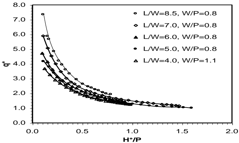
Fig. 6. Performance du P.K.Weir en fonction du ratio L/W
