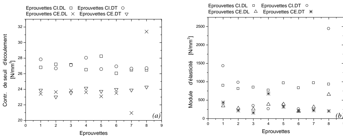
Figure 8: Evolution de \sigma_y (a) et E (b) dans la couche externe pour DL et DT.
